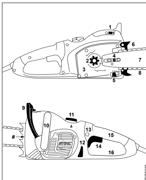
1 Сигнальная лампа электронной защиты от перегрузки
